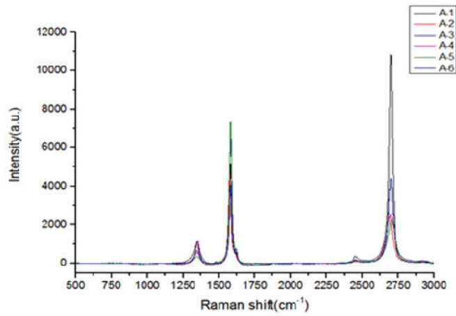
图4. 石墨烯典型拉曼光谱图
